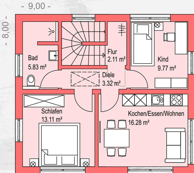
Obergeschoss
