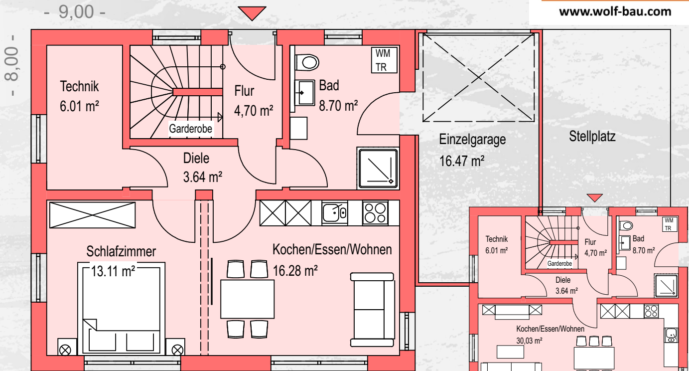
Erdgeschoss
